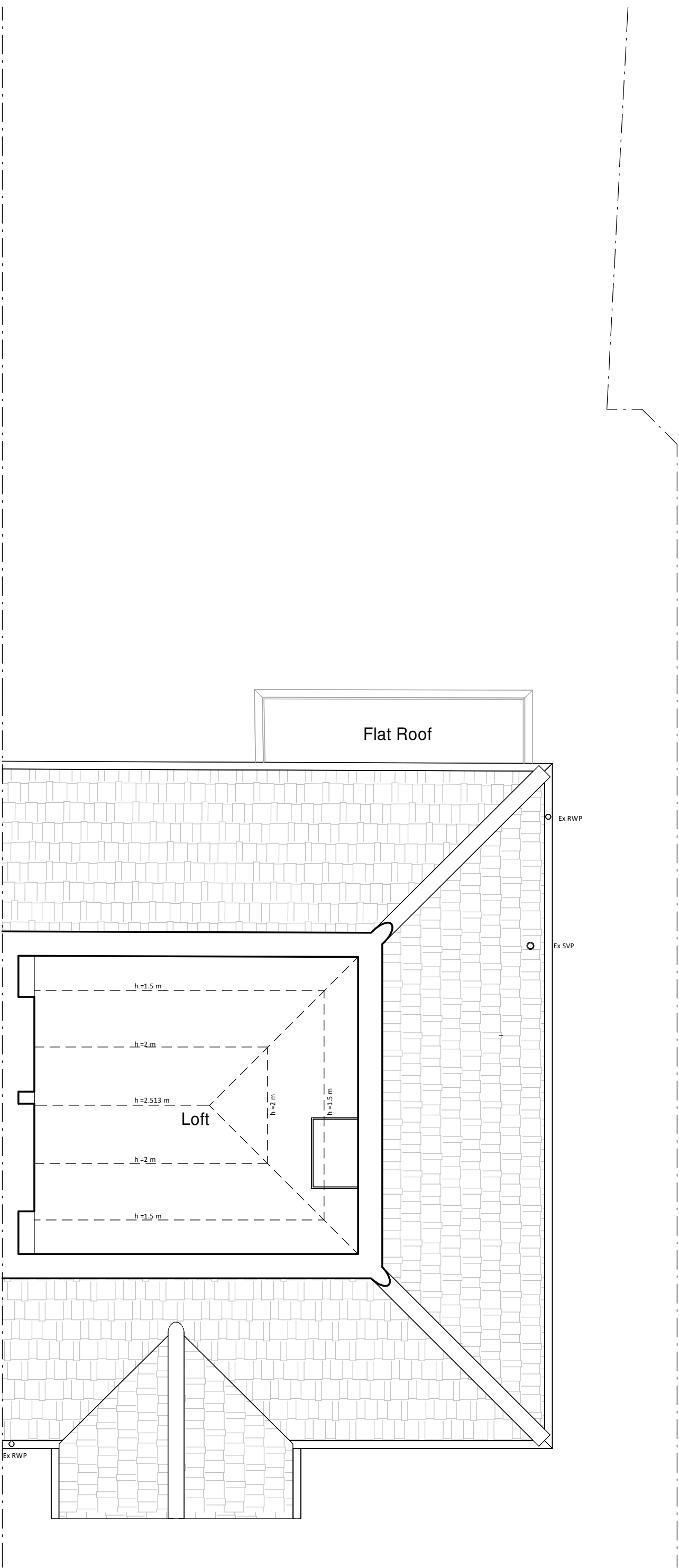
Loft Plan
